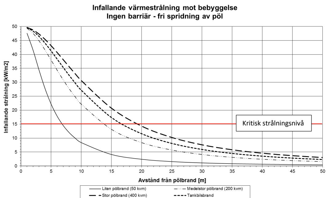
Figur B. 7. Infällande strålning som funktion av avståndet från pölbrand.
