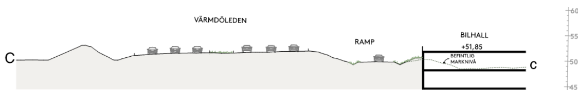
Figur 3.1. Sektion genom underbyggd markparkering och påfartsramp. Sektionen visar utsnitt C i figur 2.4 (ÅWL arkitekter, 2020-09-01).
