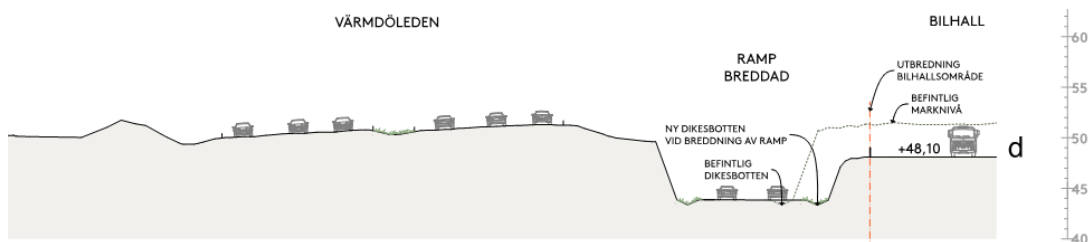
Figur 2.5. Sektion (D, längst till höger i figur 2.4) (ÅWL arkitekter, 2020-09-01).
