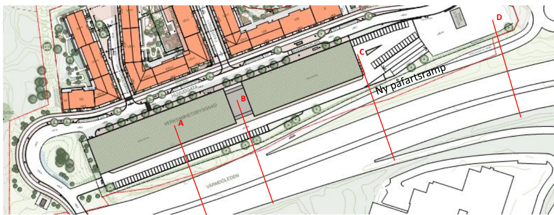
Figur 2.4. Ryssbergen situationsplan (ÅWL arkitekter, 2020-12-21).
